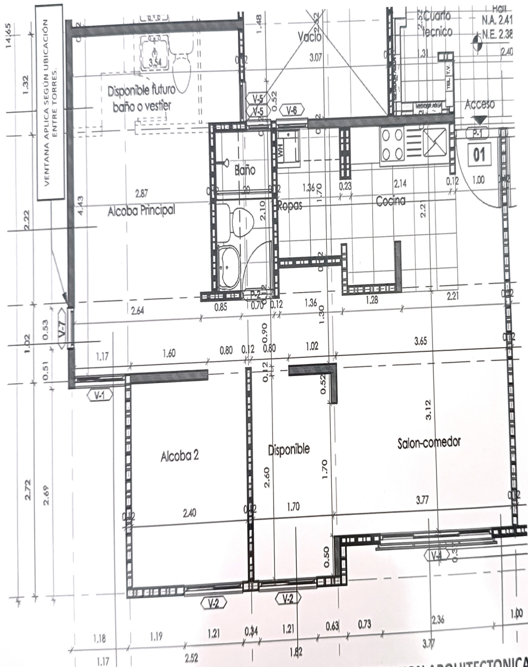
PLANTA DE DISTRIBUCION ARQUITECTONICA APTOS 201-301-401-501
