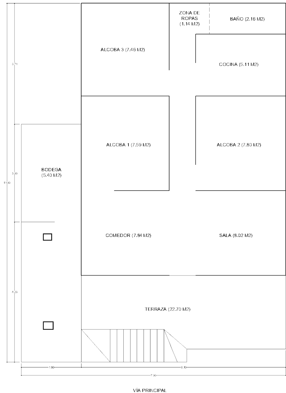
PLANTA ARQUITECTÓNICA PISO 1
