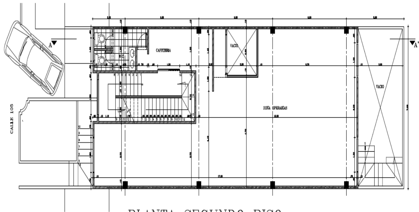
PLANTA SEGUNDO PISO
