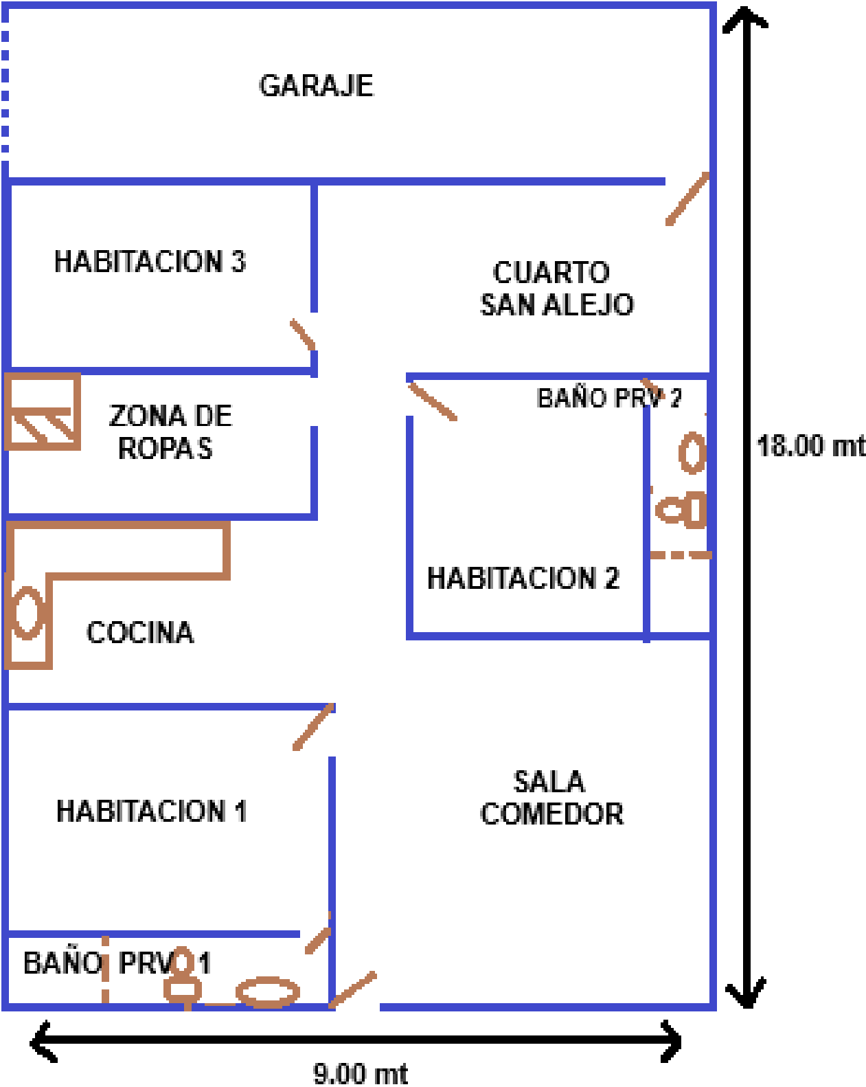
Plano
