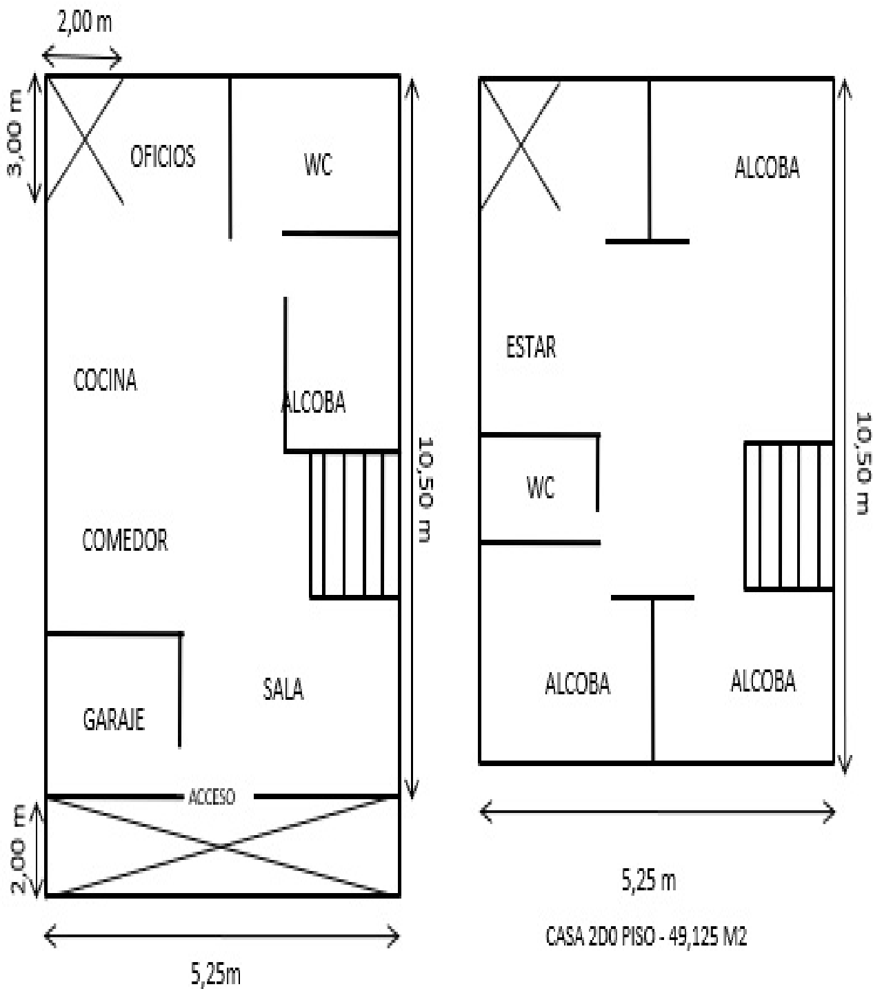
CASA 1ER PISO - 49,125 M2
