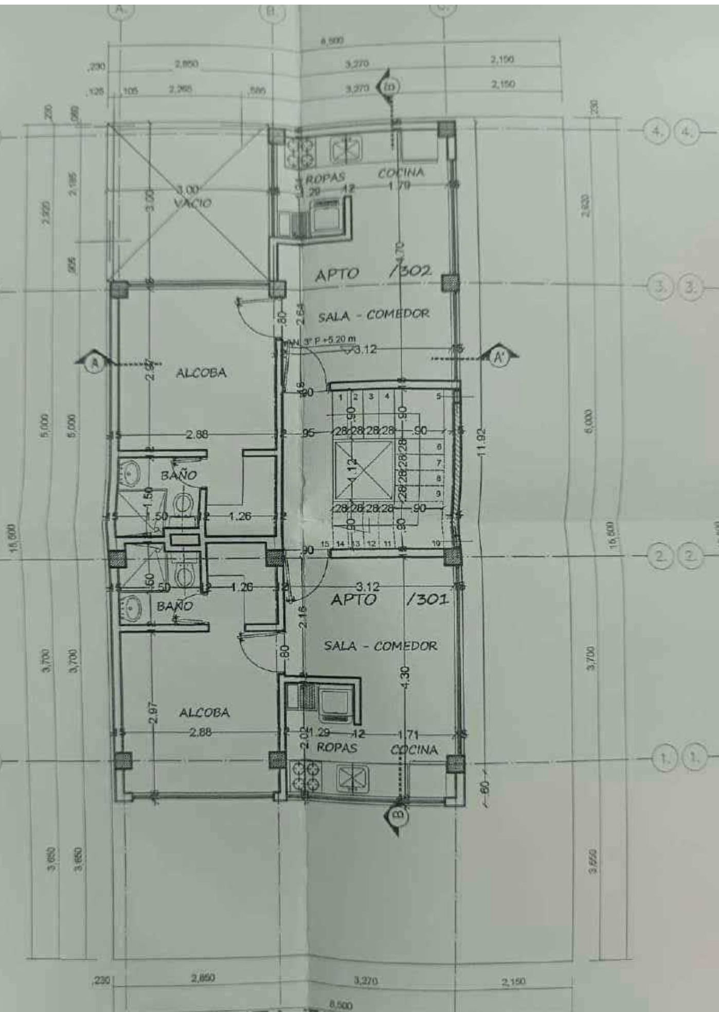
PLANTA TIPO 3° PISO
