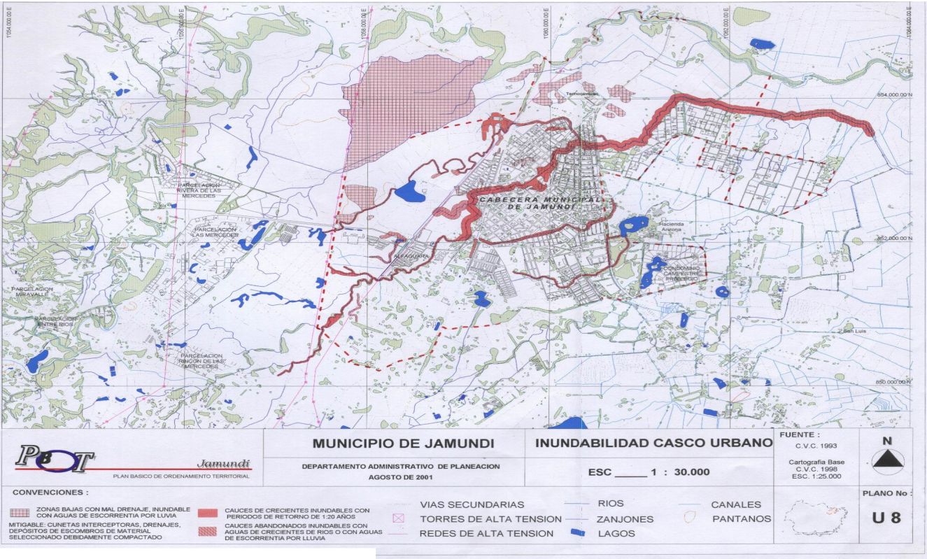
Plano Inundación
