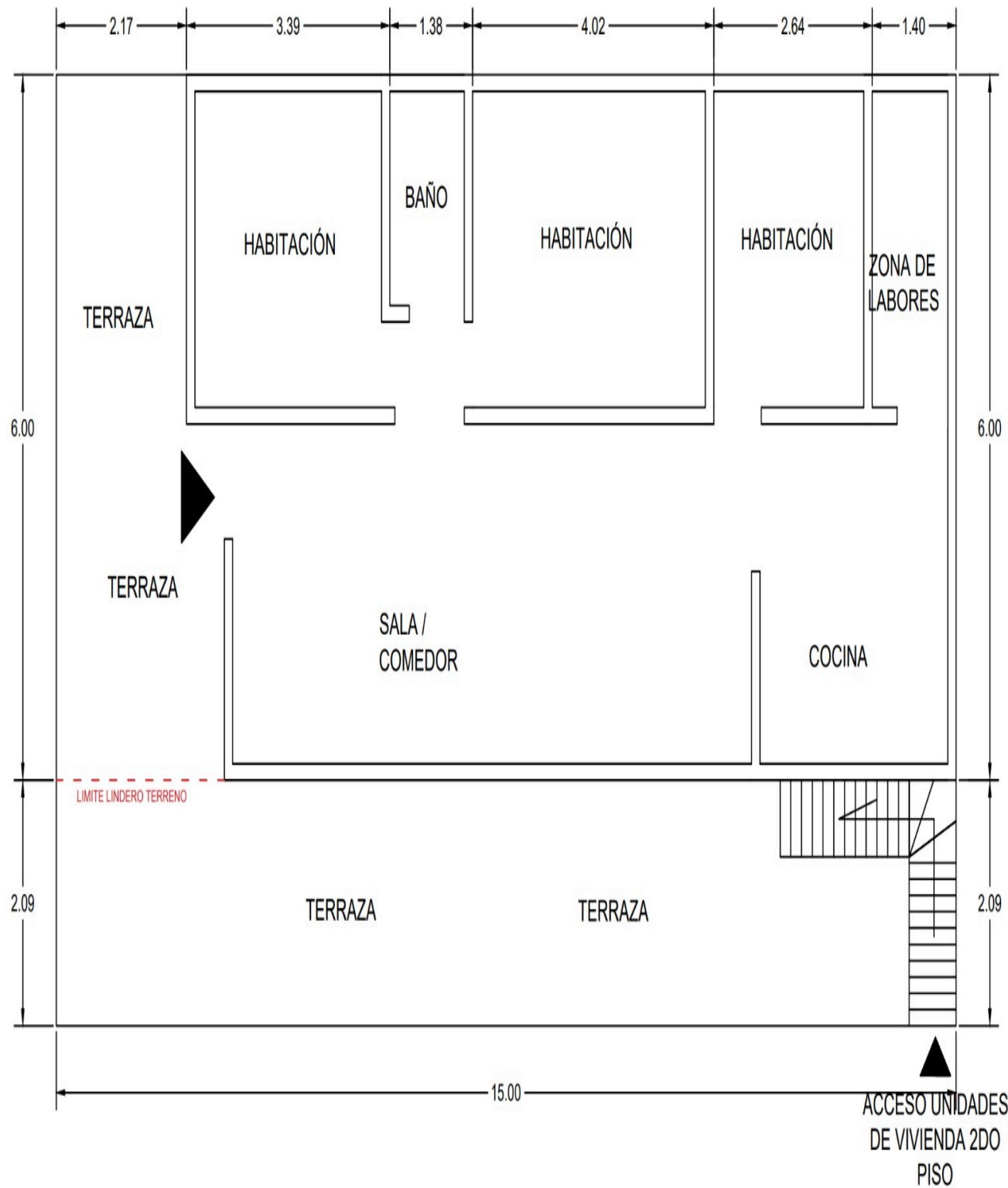
Plano
