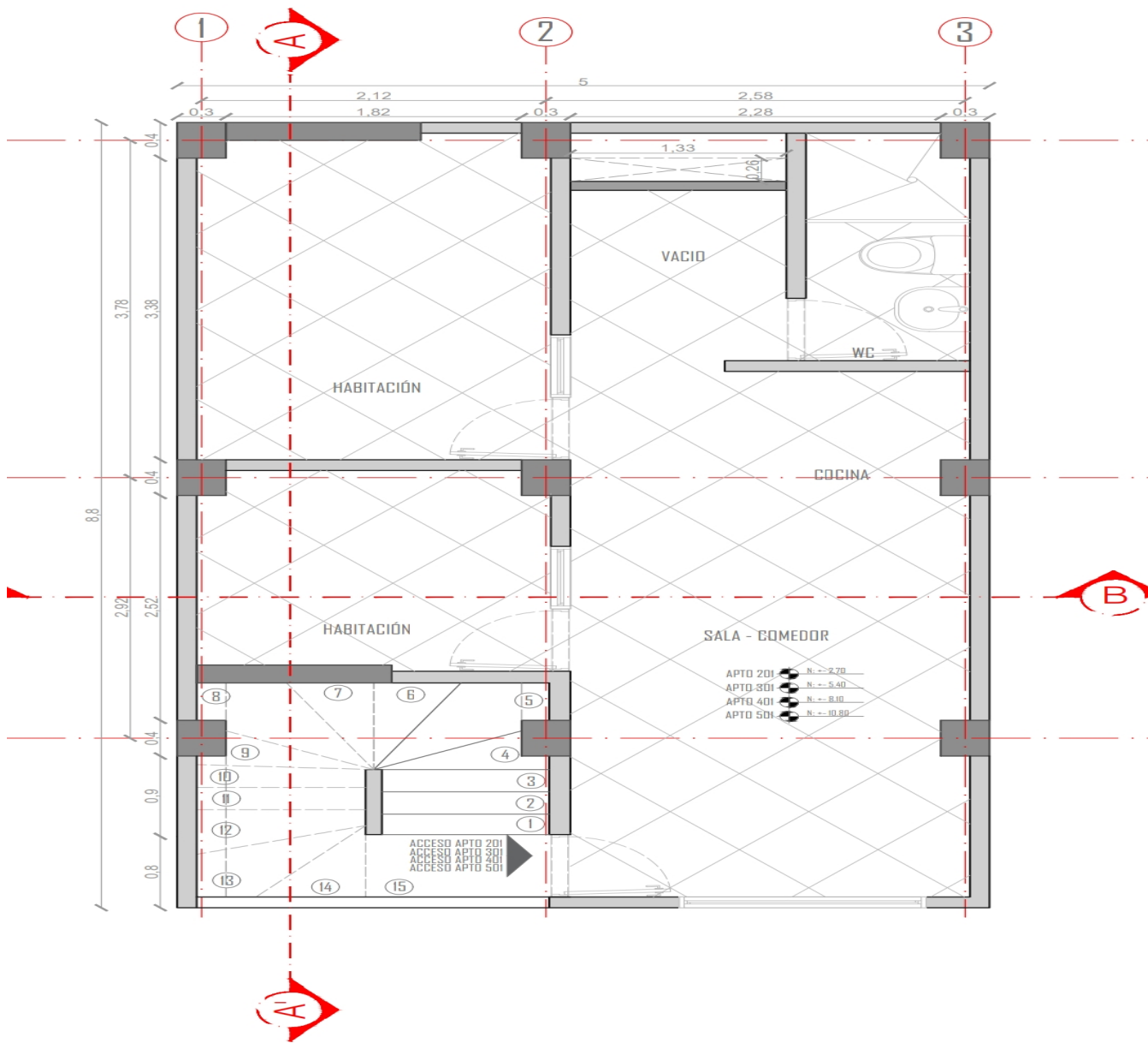
PLANTA TIPO (SEGUNDO, TERCER, CUARTO Y QUINTO PISO) N: +2.70 /N: +5.40/N: +8.10/N: +10.80 / ESC: 1:50
