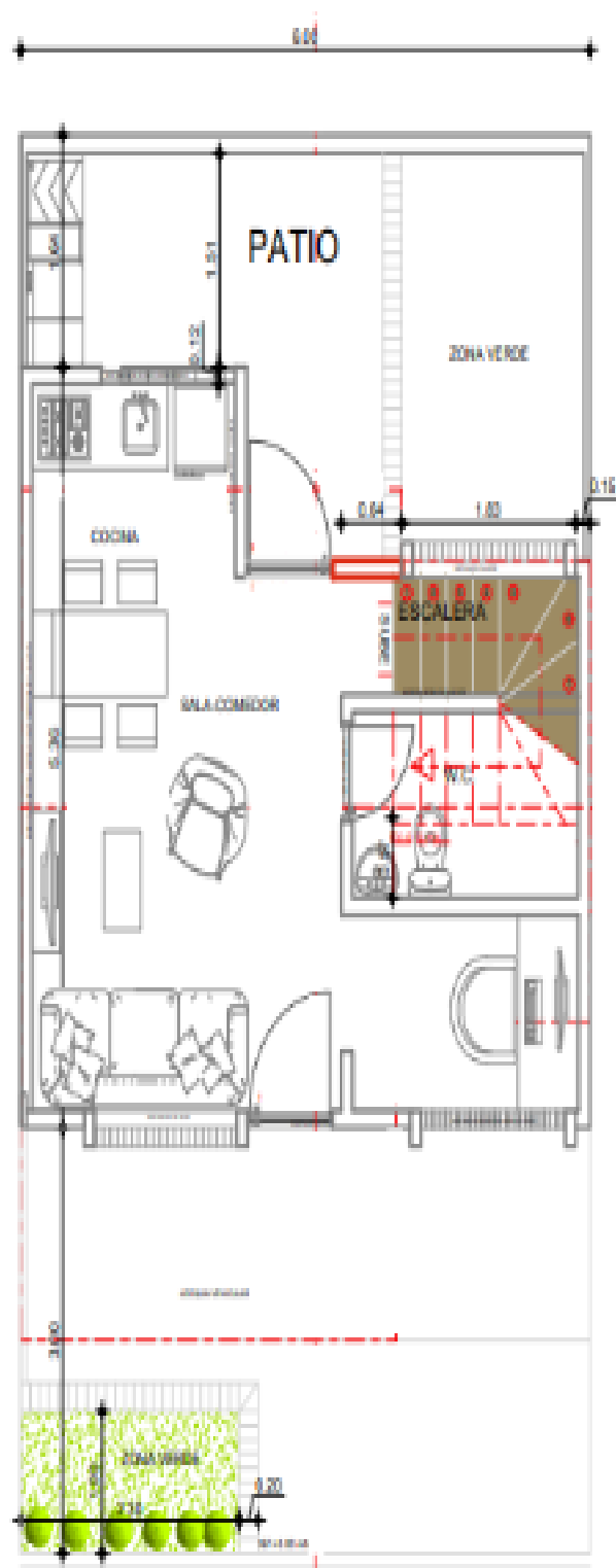
PLANTA PRIMER PISO SC: 1_50
