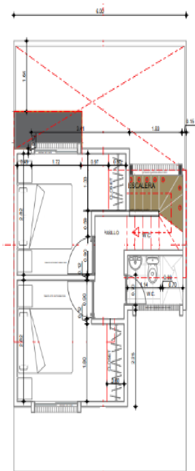
PLANTA SEGUNDO PISO SC: 1_50
