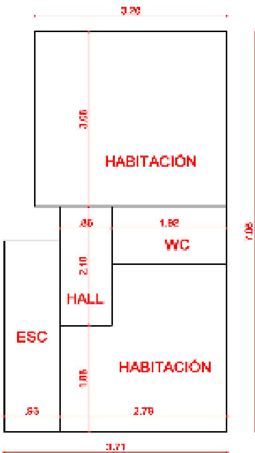
PISO 02
