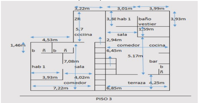
plano piso 3
