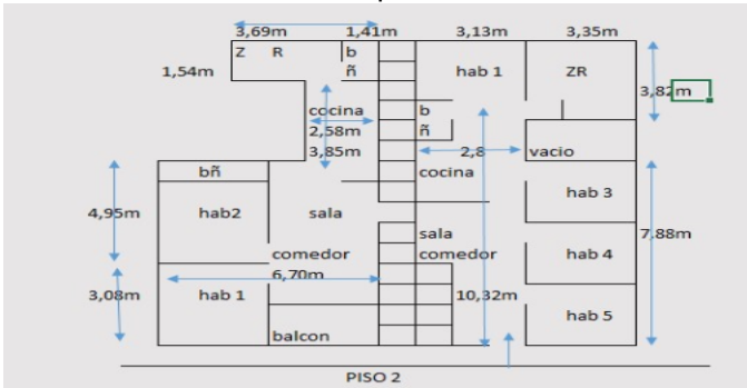
Plano piso 2
