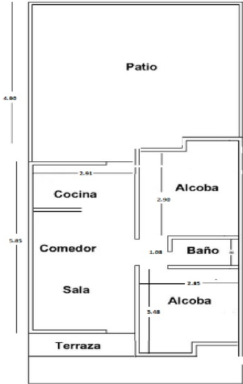
PLANTA ARQUITECTONICA
