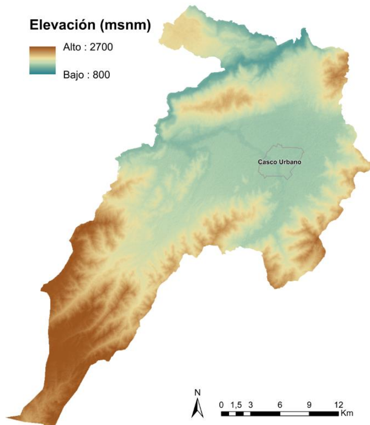
Figura 2. Elevación, en metros sobre el nivel del mar (msnm), del Municipio de Pitalito.
